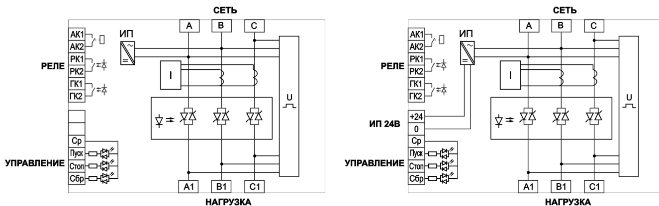
а) БСТ2-Н40, БСТ2-Н41, БСТ2-Н42
