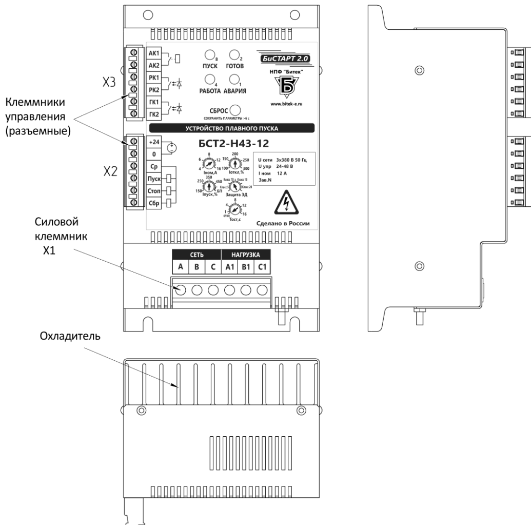
Рисунок 1 - Внешний вид пускателя БСТ2-Н43-12 (см. также Приложение А)
