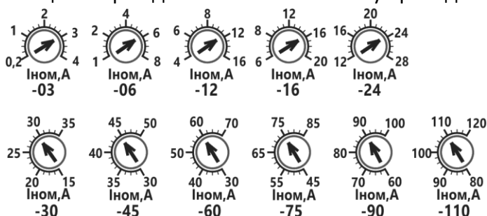
Рисунок 6 Диапазоны настройки Ином
