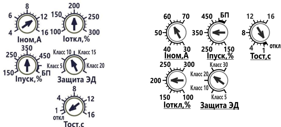
Рисунок 5 Органы настройки БСТ2-Н4
